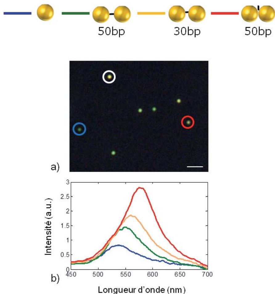
Figure 3.6 – (a) Exemple d’images en champ sombre prises par la caméra couleur (Qicam , temps d’acquisition de 500 ms). Le diffuseur entouré d’un cercle bleu représente une particule seule de 36 nm, le cercle rouge entoure la lumière diffusée par un dimère, et le cercle blanc identifie un agrégat. (b) Spectres de résonance de particules seules (courbe bleue), de dimères de 50 pb et 30 pb (courbes verte et jaune), et d’un dimère lié d’un double brin d’ADN de 50 pb perpendiculaire à l’axe principal (courbe rouge).
