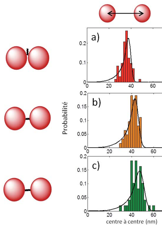
Figure 2.18 – Distributions des distances "centre à centre" a) dimère lié par un double brin de 50bp perpendiculaire b) dimère lié par un double brin de 30bp c) dimère lié par un double brin de 50bp.
