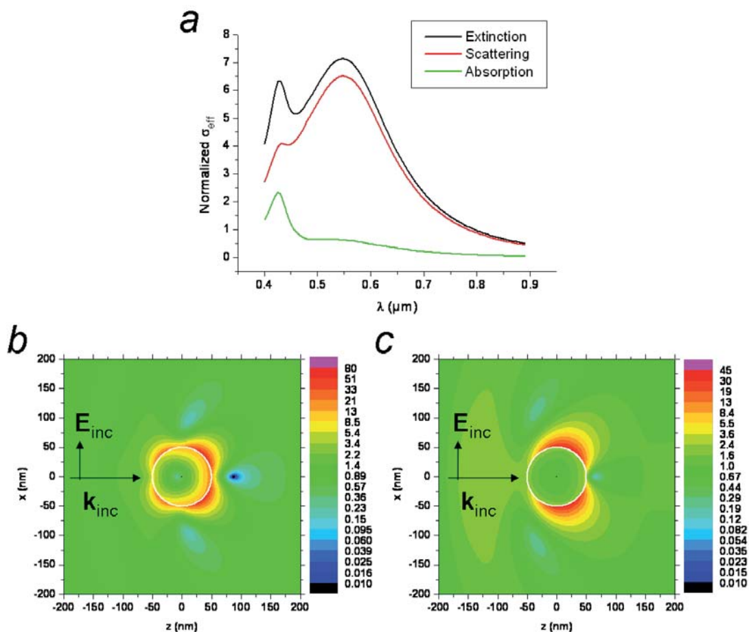
Figure 1.5 – (a) Calculs par la théorie de Mie des sections efficaces d'une particule sphérique d'argent de 100 nm de diamètre avec un indice diélectrique du milieu n_m=1.5 et de l'argent massif pour la particule. Cartes de la distribution de l'intensité calculées : longueur d'onde d'excitation \lambda = 430 \text{ nm} (b), longueur d'onde d'excitation \lambda = 550 \text{ nm} (c). Figure tirée de la thèse d'Alexis Devilez [127].
