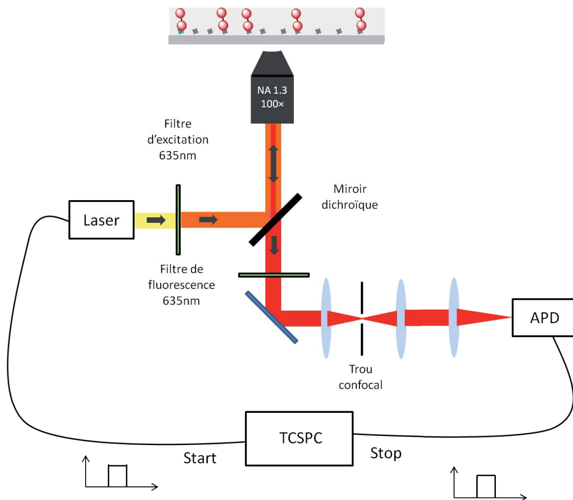
Figure 4.5 – Schéma de principe d'une expérience de mesure de temps de vie de fluorescence (TCSPC : Time Correlated Single Photon Counting, APD : Single Avalanche Photodiode).
