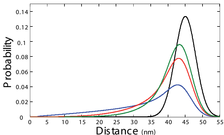
Figure 2.22 – Graphique de comparaison entre la distribution gaussienne D_l (courbe noire) et la distribution de projection D_{\tilde{l}}(\tilde{l}) pour D_\theta(\theta) = \frac{1}{\pi} (courbe bleue), D_\theta(\theta) = \frac{2}{\pi} \sin^2(\theta) (courbe rouge) et D_\theta(\theta) = \frac{8}{3\pi} \sin^4(\theta) (courbe verte)
