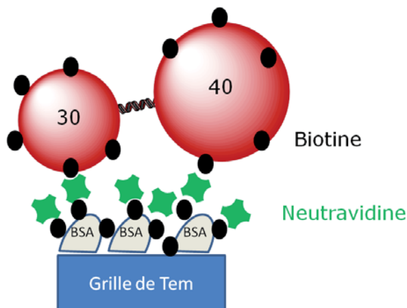
Figure 2.13 – Fonctionnalisation des grilles de carbone avec deux couches de protéines. Les particules sont enrobées de PEG biotinyté qui se lie à la Neutravidine déposée sur les grilles de TEM.
