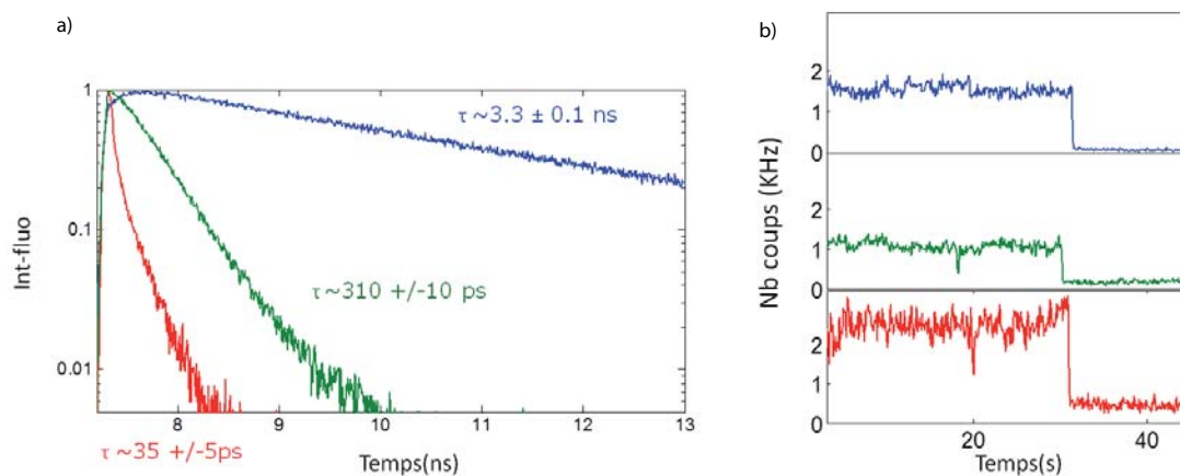
Figure 4.7 – (a) temps de vie de fluorescence typique (b) signal de fluorescence (moyenné sur 100 ms) de molécules d'ATTO647N pour un émetteur isolé (courbe bleue, temps de vie estimé 3.2 \pm 0.150 \text{ ns} ), NPAu seule fonctionnalisée avec un brin d'ADN de 50 bp (courbe verte, temps de vie estimé 310 \pm 10 \text{ ps} ), dimère de 30 pb (courbe rouge, temps de vie estimé 35 \pm 5 \text{ ps} ).
